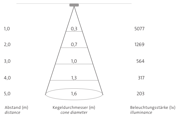
medium 24° + Wabenraster schwarz
