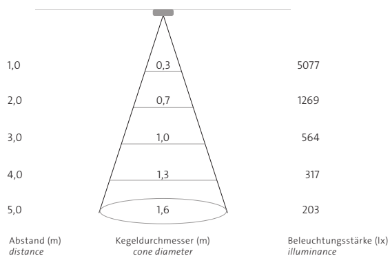
medium 24° + Wabenraster schwarz
