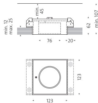
Deckenausschnitt: 125 × 125 mm
